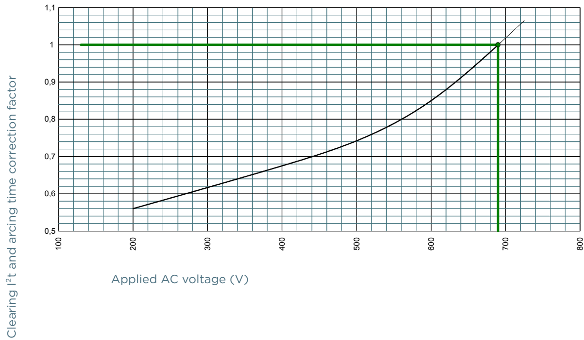
Size 73 aR 690V
